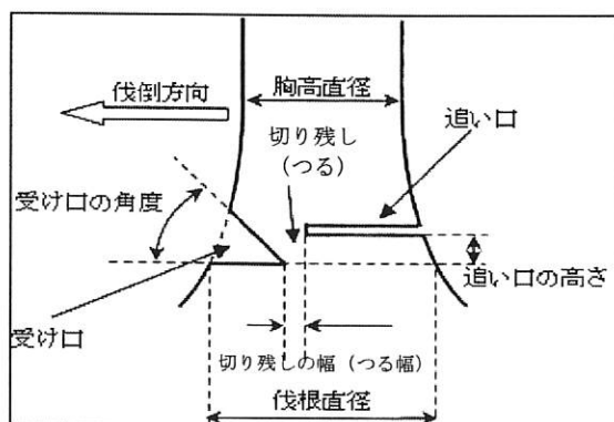
図1 受け口、追い口及び切り残し(つる)の関係
